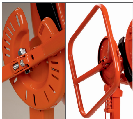
Ergonomisches Handrad mit Multirastscheibe oder Scheibenbremse mit Fußbedienung*.
