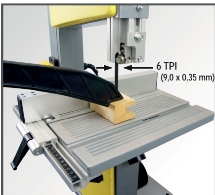
Präzises und sicheres Arbeiten dank Parallelanschlag, 3-Rollen Sägebandführung & Schiebestock.
