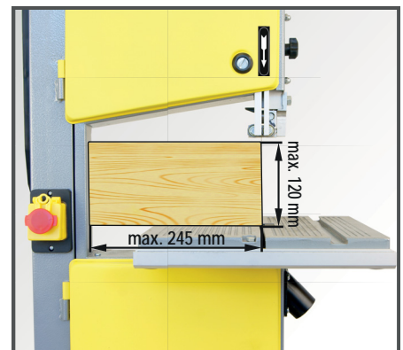
Ein-/Ausschalter mit Wiederanlaufsicherung für mehr Sicherheit. Werkstückgröße max. 245x120 mm.
