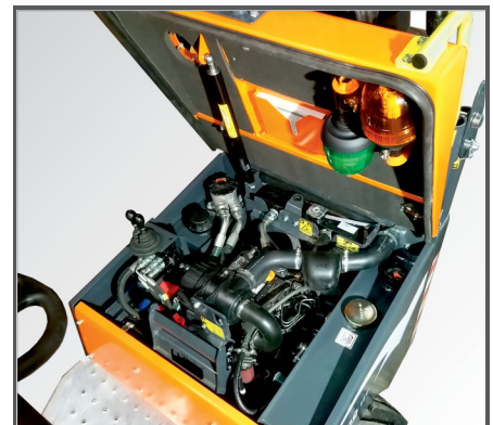
Guter und übersichtlicher Zugang, mit selbstsichernder Gasdruckfeder, zu den wichtigsten Bauteilen des bewährten YANMAR 3TNY76 Dieselmotor.
