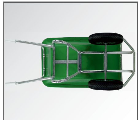
Robuster, 1-teiliger, verzinkter Stahlrohrrahmen. An 8 Punkten mit der Mulde verschraubt.
