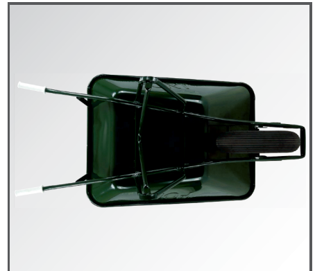
Stabiler, 1-teiliger, pulverbeschichteter Stahl-Ovalrohrrahmen mit Verstärkungsstreben und Verschleißkufen. Rahmen & Mulde komplett verschweiß.
