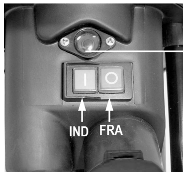
Tilbageknop (Motorvæn)
