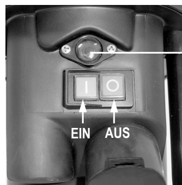
Rückstellknopf (Motorschutz)
