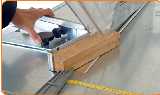
Quer- und Gehrungsanschlag mit Keilschneidlehre
