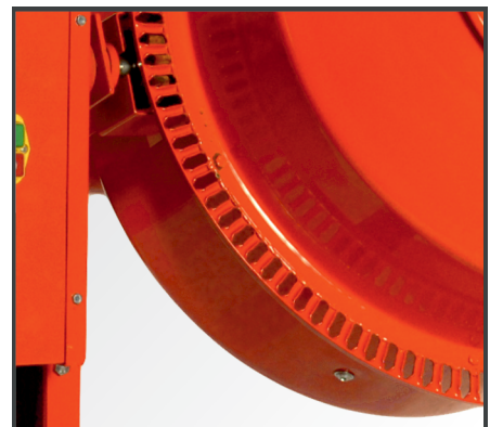
Bruchsicherer Zahnkranz aus Stahlblech, Antriebsritzel aus abriebfestem Grauguss sowie Pulverbeschichtung für eine lange Lebensdauer.
