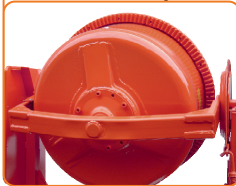
stabile Trommellagerung mit zusätzlichem Verstärkungskreuz
