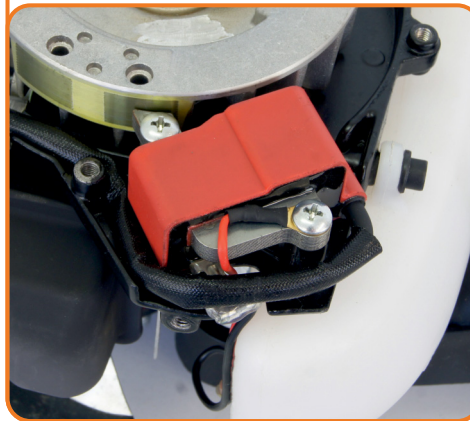
elektronische Zündung
