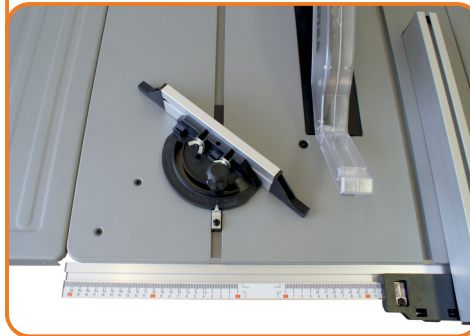
Längsanschlag und Queranschlag
