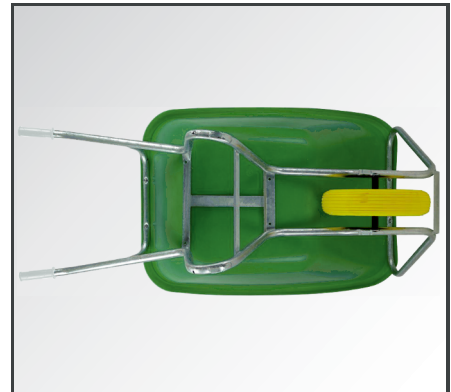
Robuster, 1-teiliger, verzinkter Stahlrohrrahmen. An 8 Punkten mit der Mulde verschraubt. Abb. mit pannensicherem Flex Pro Rad.
