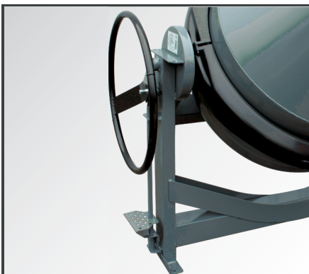
Großes Handrad mit Schwenkgetriebe und Fußpedal für die leichte Trommelverstellung. Verstärktes Gestell für mehr Stabilität.
